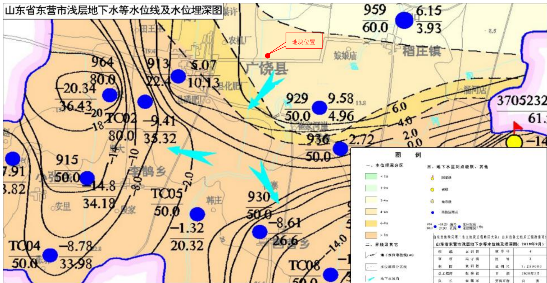
图 3.2-4 区域地下水等水位线及埋深图
