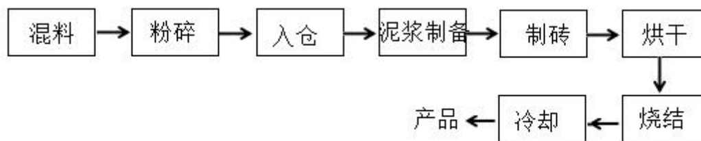
图 4.5-2 砖厂企业工艺流程图
