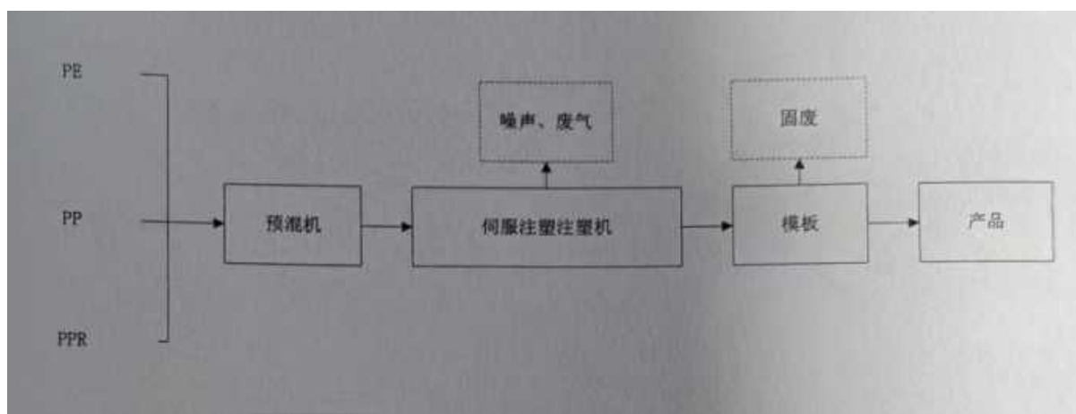
图 4.6-2 注塑工艺流程图
