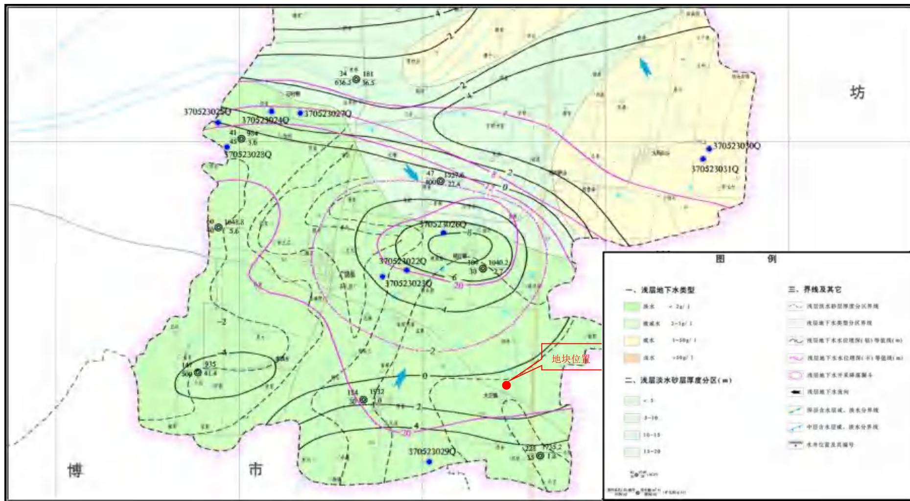
图 3.2-3 区域水文地质图
