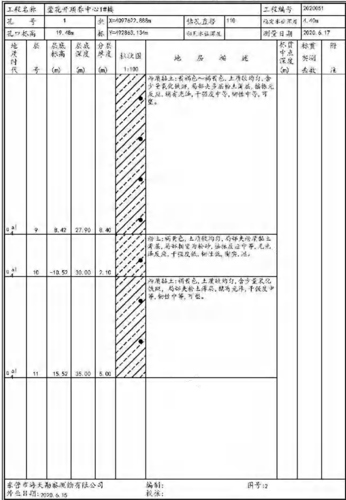
图 3.2-7 工程地质勘察柱状图
